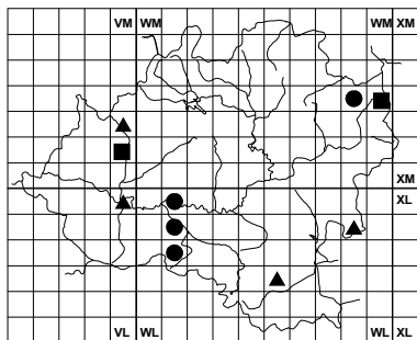
Mercurialis huetii
