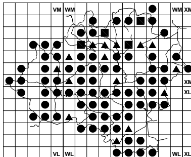
Quercus faginea
