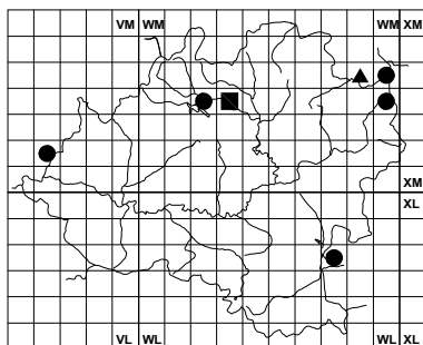
Quercus coccifera
