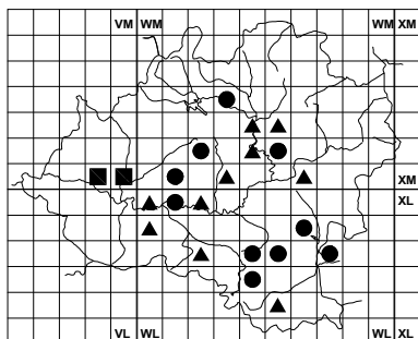
Silene conoidea
