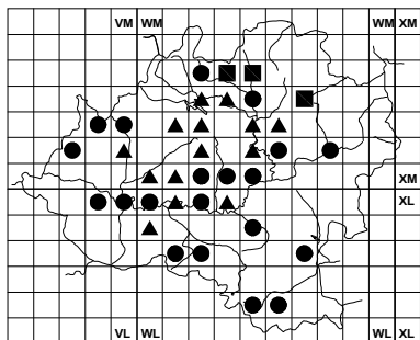
Silene colorata
