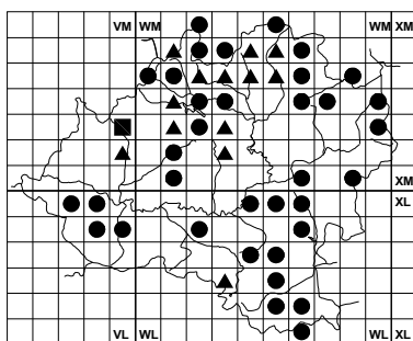
Silene nutans
