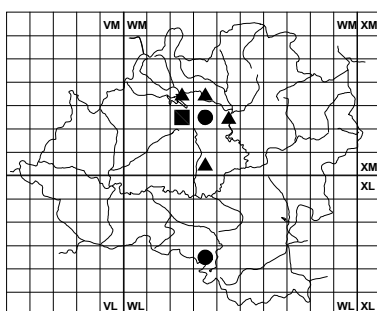
Silene gallica
