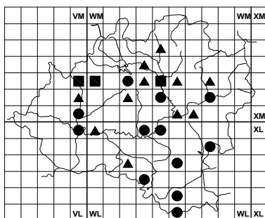
Silene conica
