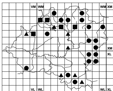
Silene latifolia
