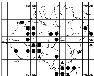
Silene mellifera
