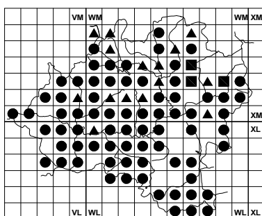
Silene legionensis
