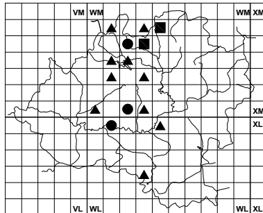
Myosotis persoonii
