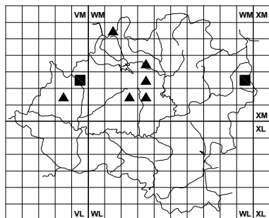
Buglossoides incrassata
