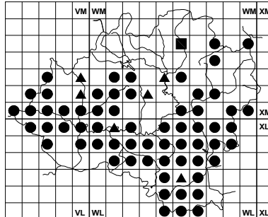
Lithodora fruticosa
