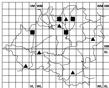
Myosotis arvensis
