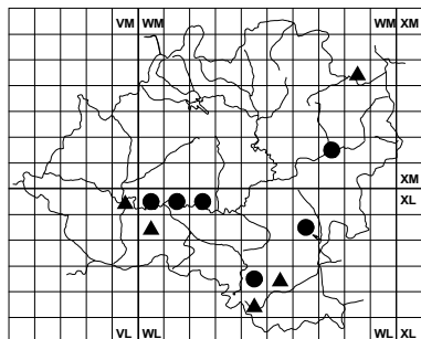
Echium asperrimum
