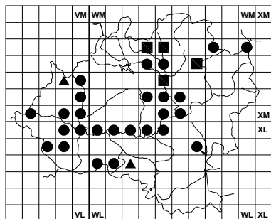
Lithospermum officinale
