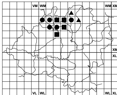
Cynoglossum officinale
