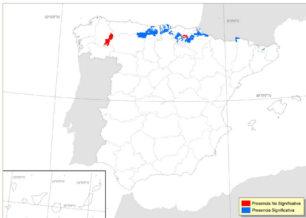
Figura 1.2 Lugares de Interés Comunitario en que está presente el tipo de hábitat 9160. Datos de los formularios normalizados de datos de la red Natura 2000, enero de 2006.
