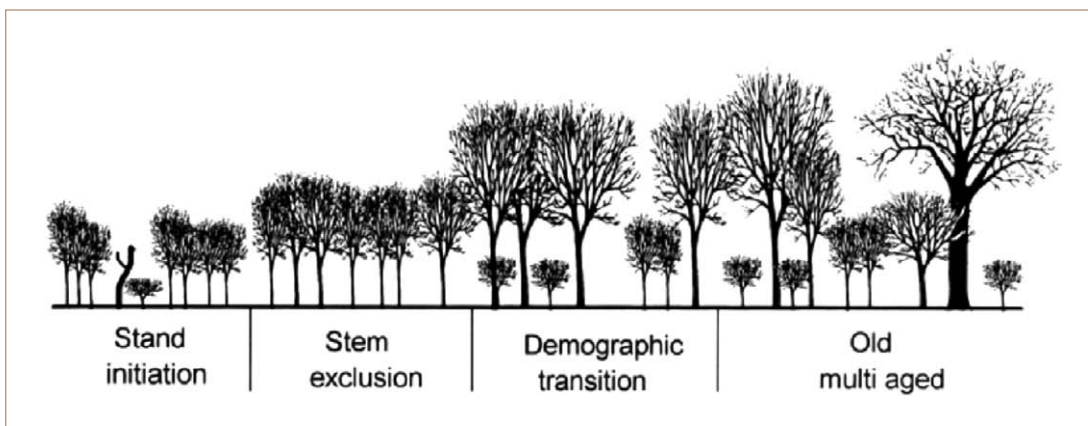
Figura 3.1 Estados sucesionales (Frelich, 2002).
