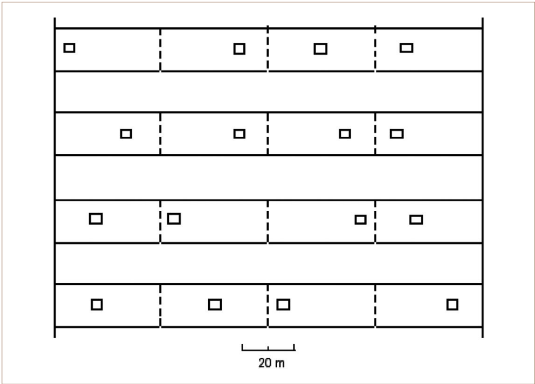
Figura 3.4 Franjas de muestreo de la madera muerta.
