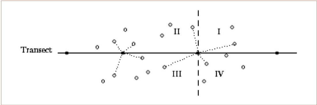
Figura 3.3 Método de los cuartos centrados en un punto.
