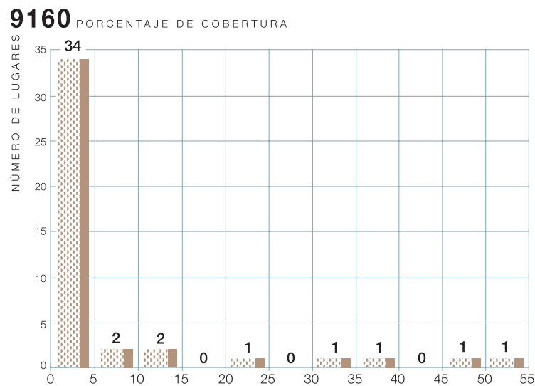
Figura 1.3 Frecuencia de cobertura del tipo de hábitat 9160 en LIC. La variable denominada porcentaje de cobertura expresa la superficie que ocupa un tipo de hábitat con respecto a la superficie total de un determinado LIC.
