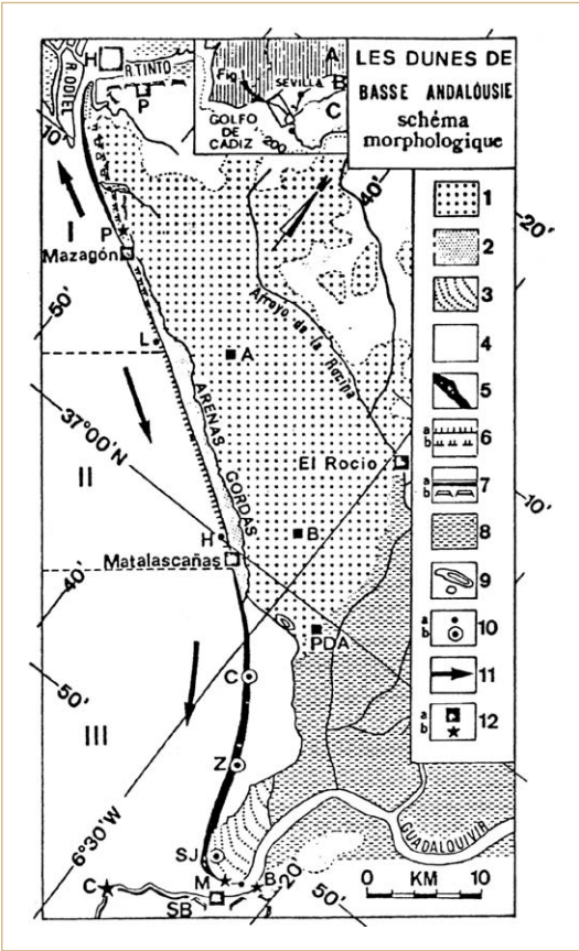
Figura 4.2 Mapa geomorfológico general del sistema de dunas de Doñana (Vanney et al. , 1979).
