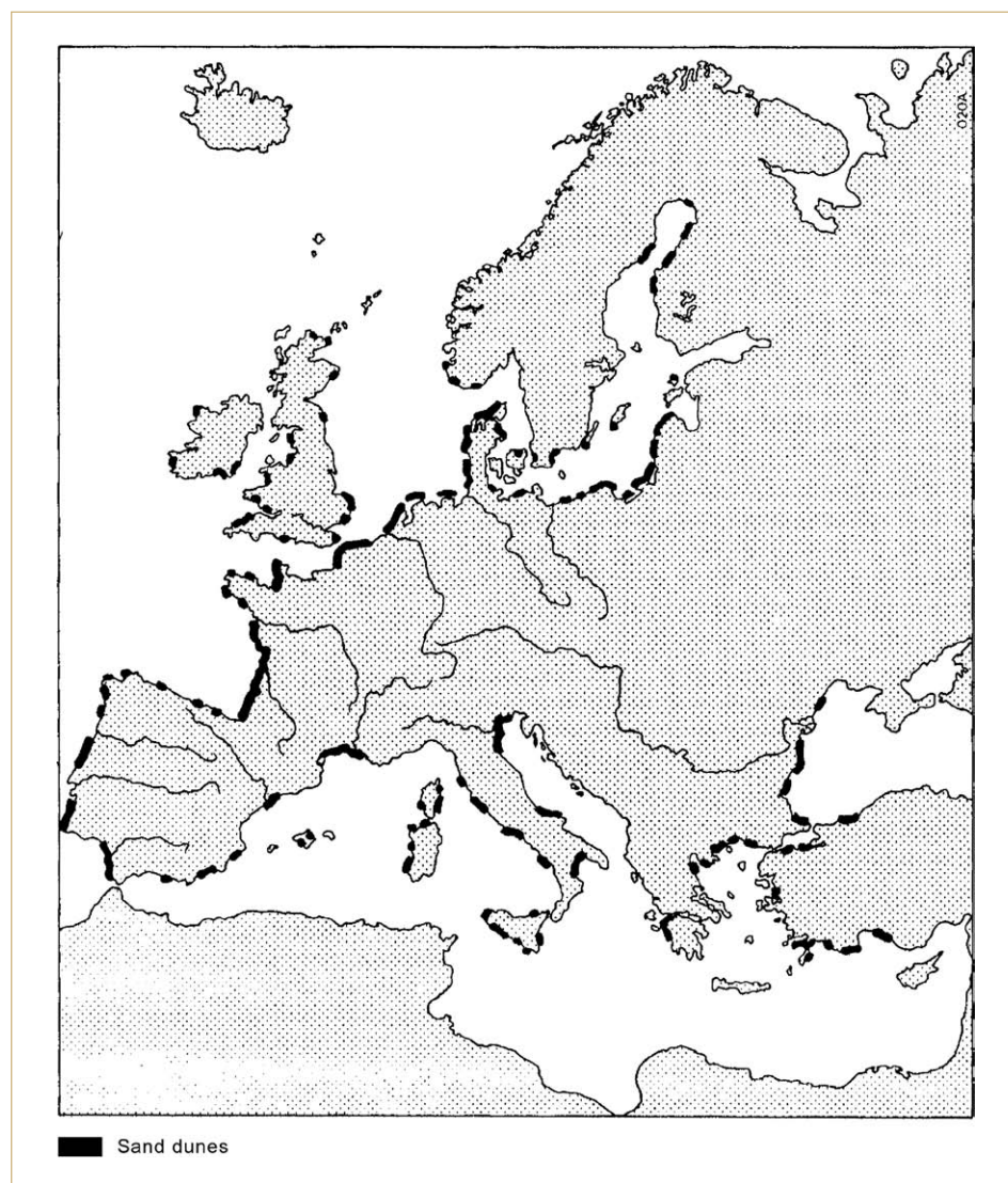
Figura 2.1 Distribución de dunas costeras en Europa (Géhu, 1985).
